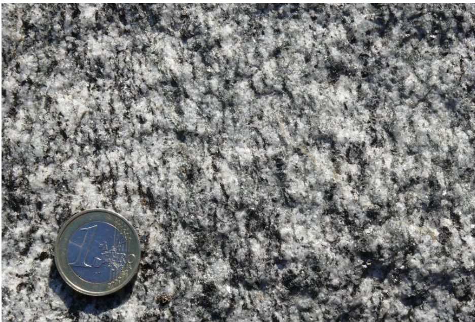
Folierter Flasergneis aus dem Steinbruch Steinach
