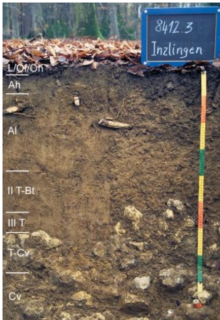
Mäßig tief entwickelte Terra fusca-Parabraunerde aus umgelagertem Lösslehm (Deck- über Mittellage) auf Karbonatgesteinszersatz des Oberen Muschelkalks (Z73)
