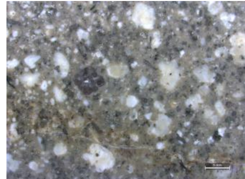
Feinkristalline Grundmasse des Granitporphyrs mit Einsprenglingen
