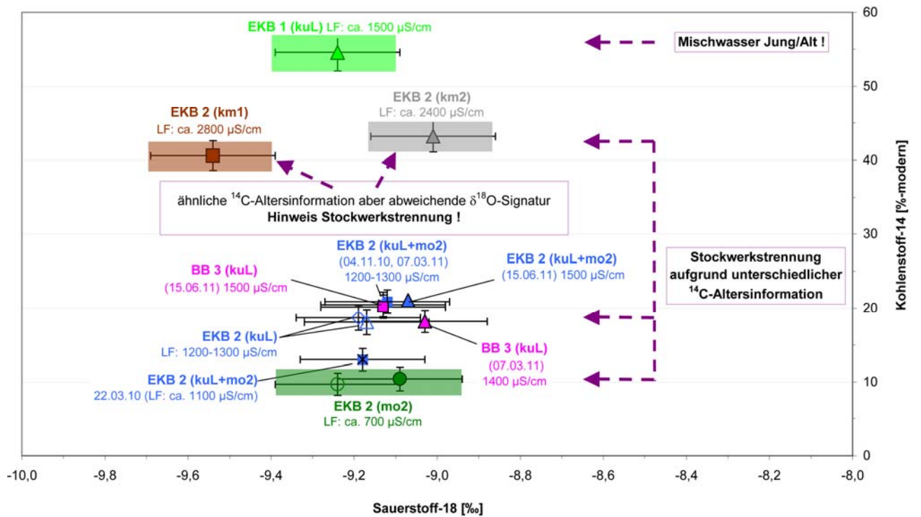
Abb. 5.7: Korrelation ^{18}\text{O}/^{14}\text{C} -Gehalte (Grafik: Hydroisotop, Emmendingen, kuL: Erfurt-Formation (kuE), mo2: Meißner-Formation (moM)).
