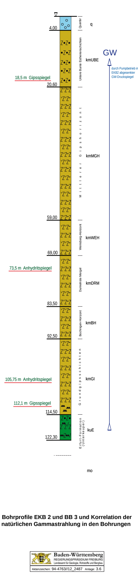
Bohrprofil BB 3
