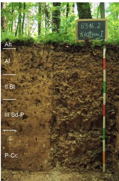
Mäßig tief entwickelte pseudovergleyte Pelosol-Parabraunerde aus lösslehmreichen Fließerden auf junggrüzeitlichen Seeablagerungen
