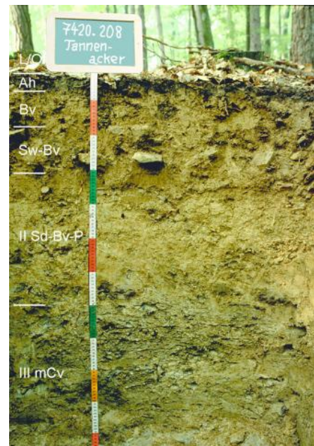
Mäßig tief entwickelter Pseudogley-Braunerde-Pelosol aus geringmächtiger lösslehmhaltiger Fließerde über tonreicher Schwarzhura-Fließerde (n5)
