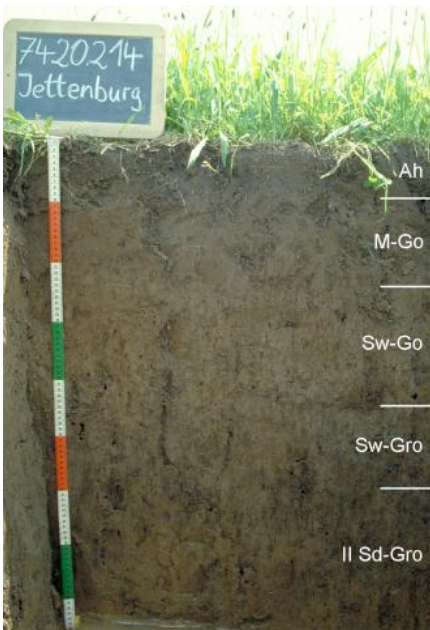
Kolluvium-Gley, pseudovergleyt, aus holozänen Abschwemmassen über Lösslehm (n30)
