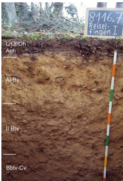
Mäßig tief entwickelte podsolige Parabraunerde-Braunerde aus lösslehmreicher Fließberde über wärmzeitlichen Flussschottern
