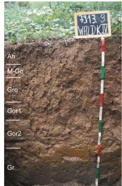
Auengley aus holozänem Auensediment (a7)
